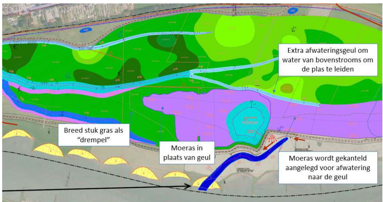
Figuur 1: Aanpassingen in ontwerp Elster Buitenwaarden t.b.v. hydrologische isolatie plas.
